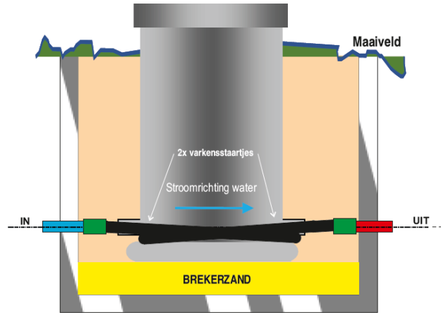
TEKENING 3: DOORSNEDE WERKPUT MET GEPLAATSTE WATERMETERPUT
